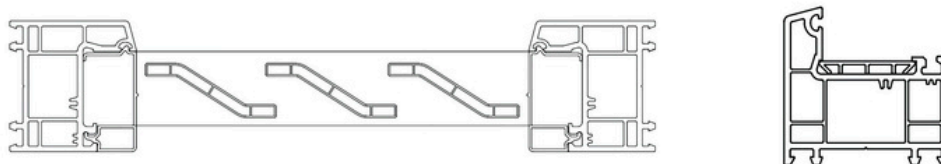
PENGUNAAN RP 45, JALUSI, DAN FL 36
