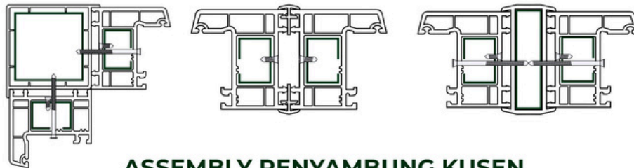
ASSEMBLY PENYAMBUNG KUSEN
